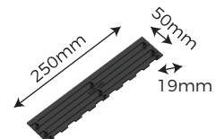
EasyDRAIN™ Edge Heel Friendly Insert EI code: 83230
