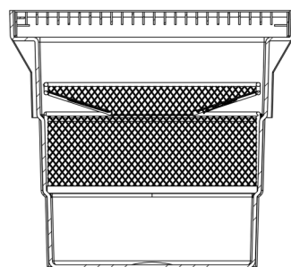
SECTION B-B SCALE 1 : 6
